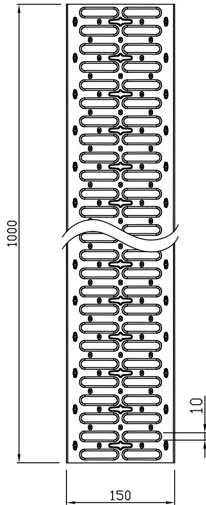
평면도 scale : None
