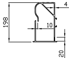
정면도 scale : None
