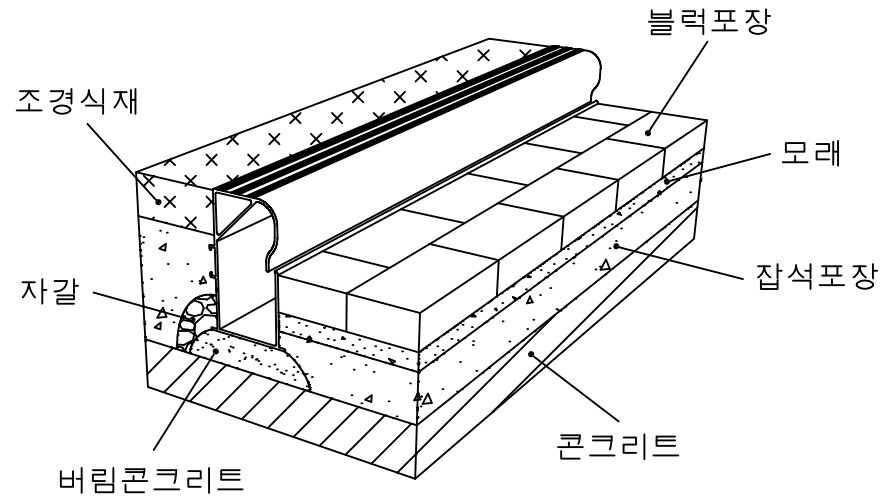
설치예시도 scale : None
